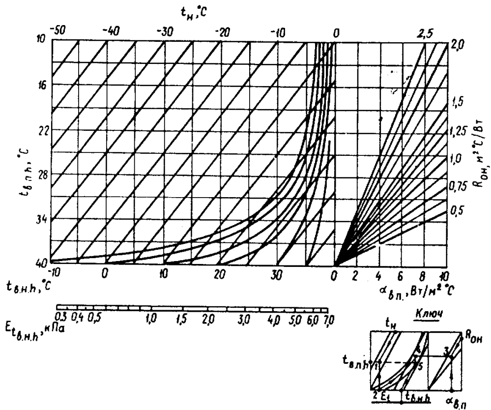
Рис. 3. Номограмма для нахождения температуры наружной поверхности воздушной прослойки t_{вн.н}, ^\circ\text{C} и максимальной упругости водяного пара воздуха E_{т.в.н.н}, \text{кПа}
