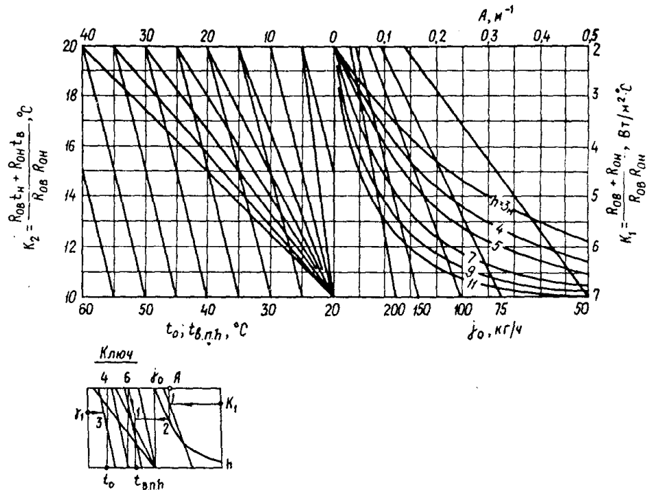
Рис. 2. Номограмма для нахождения температуры воздуха, поступающего в вентилируемую прослойку стены t_0 , °С
