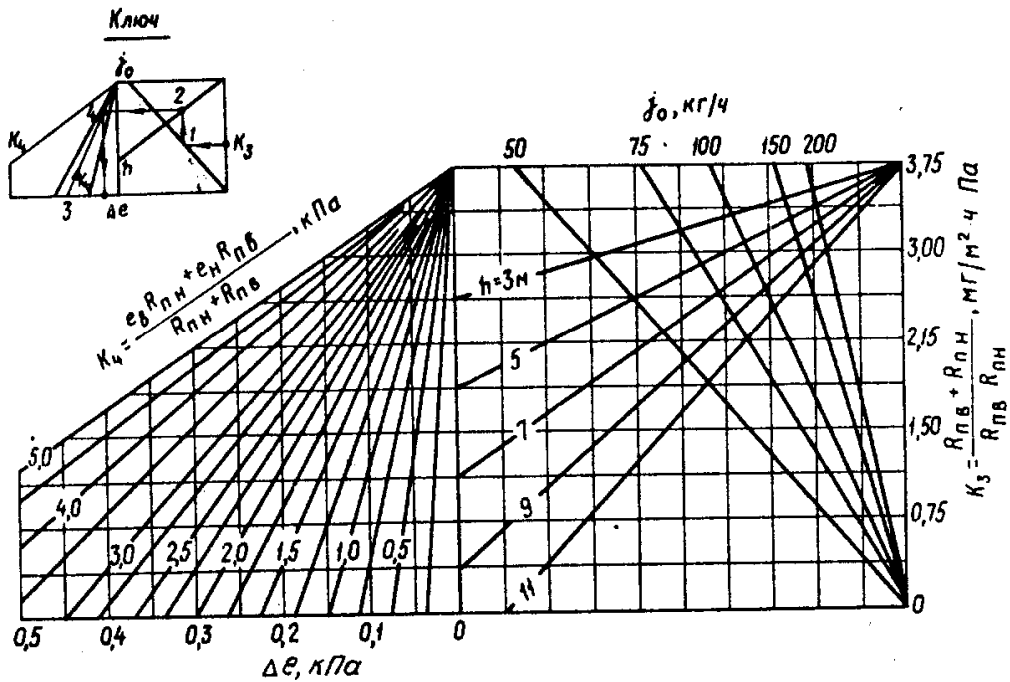
Рис. 4. Номограмма для нахождения изменения действительной упругости водяного пара воздуха вентилируемой прослойки \Delta l, \text{кПа}
