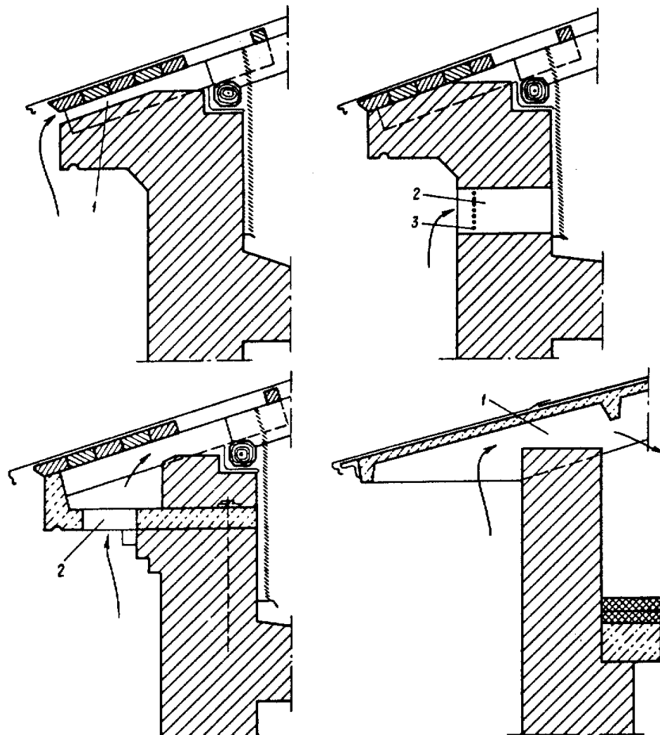
Рис. 1. Схемы чердачных крыш с расположением вентиляционных отверстий: а - под свесом кровли и в коньке крыши; б - в карнизной части стены и в коньке крыши; 1 - щелевидной формы; 2 - прямоугольной формы
